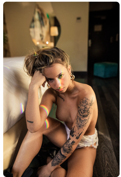
ComfyUI.
